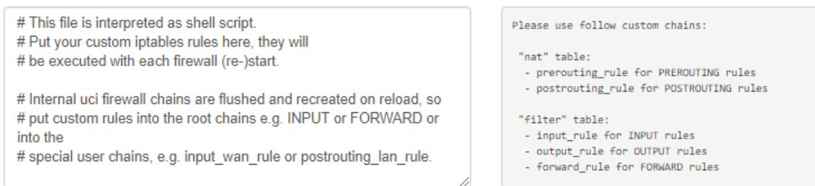
Рис. 30. Вкладка Services, раздел Firewall, настройки User Firewall Rules
