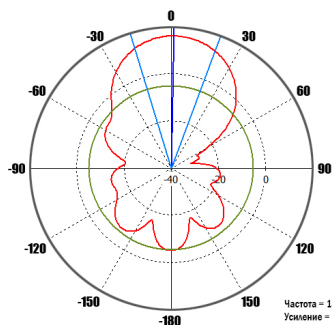
Частота = 1800 МГц Усиление = 15,7 дБи Угол раскрытия по уровню -3 дБ = 19,7° Уровень боковых лепестков = -10,2 дБ
