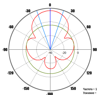
Частота = 1800 МГц Усиление = 15,9 дБи Угол раскрытия по уровню -3 дБ = 21,4° Уровень боковых лепестков = -12,3 дБ
