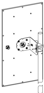
Рисунок 2 – Монтаж антенны на мачте
