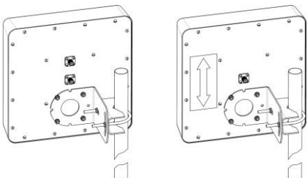
Рисунок 2 – монтаж антенны на мачте
